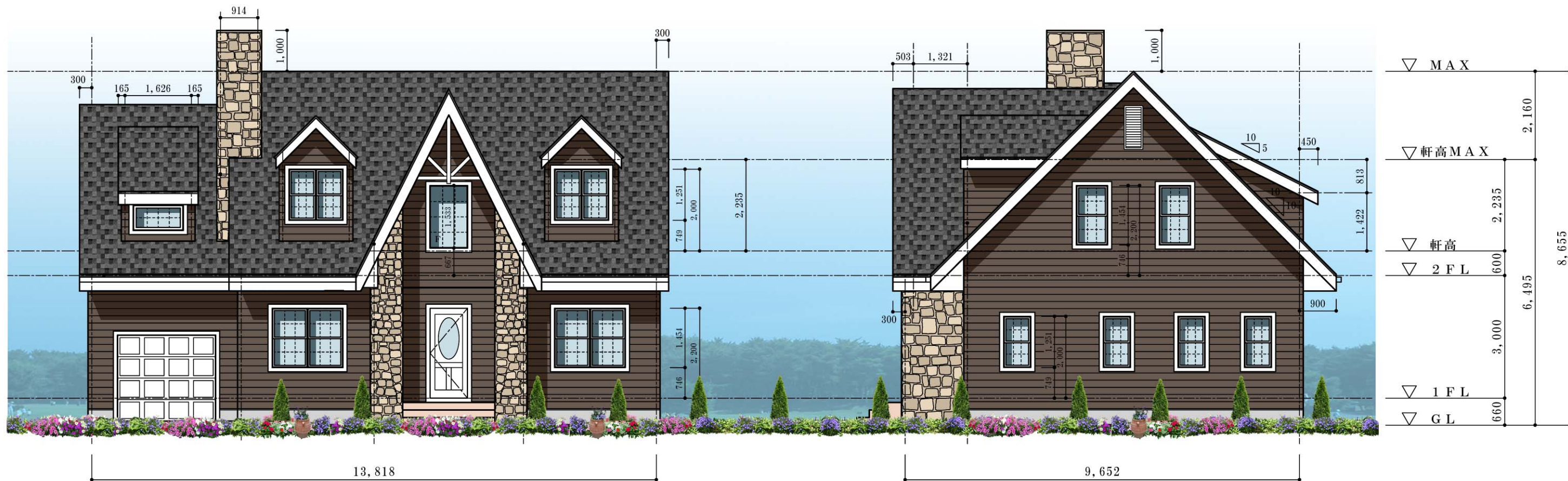
東立面图 1/100
